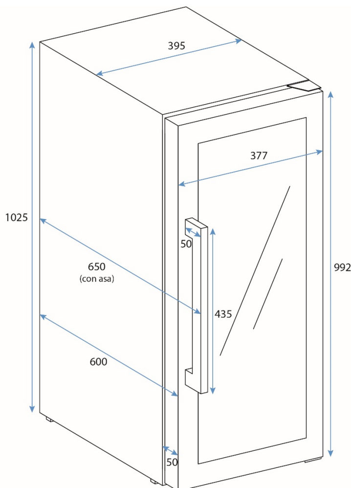
Figura: Dimemsionamiento
