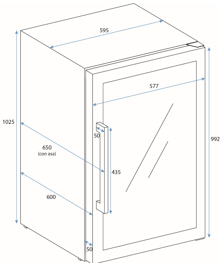
Figura: Dimemsionamiento
